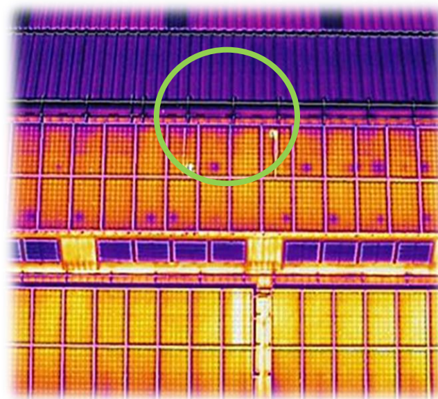
太陽光電模組檢測影像
